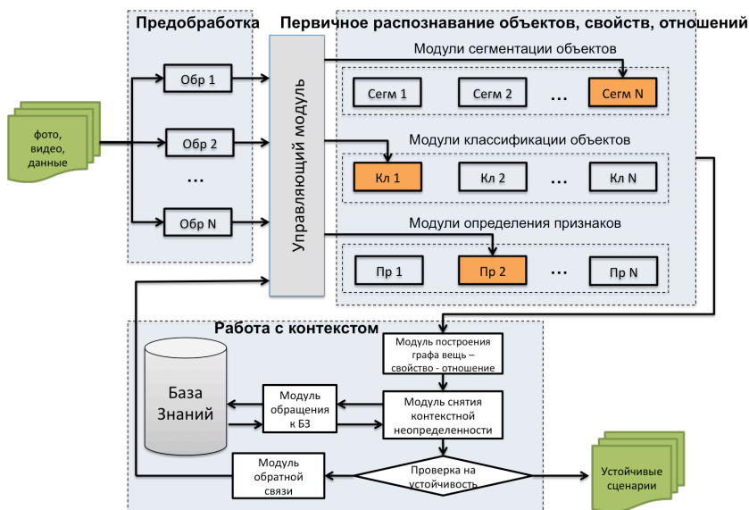
Рис. 1. Модульная схема системы
