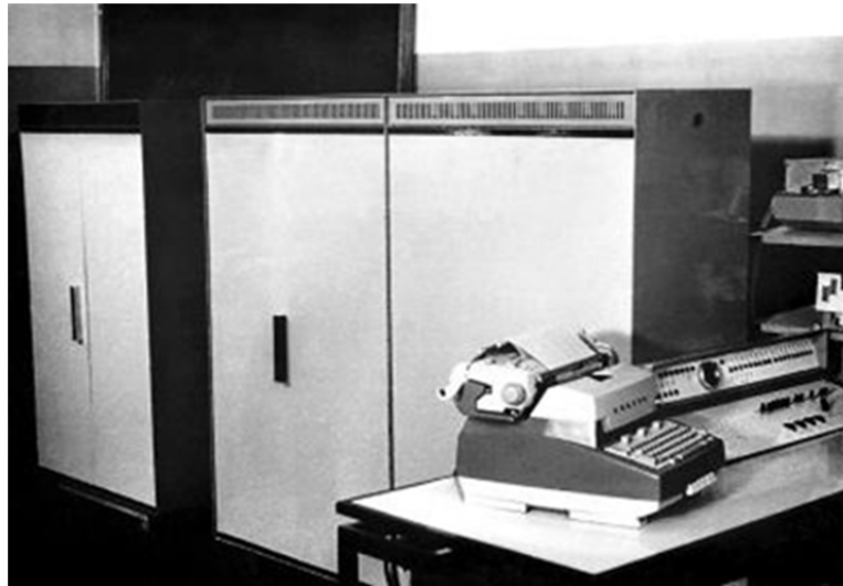
Рис. 2. ЭВМ «Сетунь 70»
